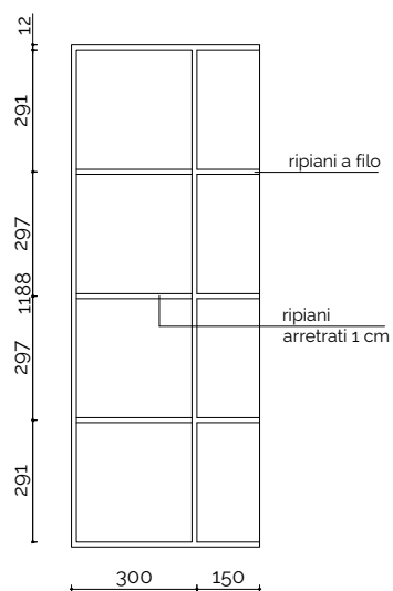
prospetto anta aperta
