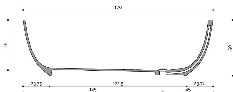
sezione
